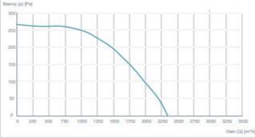
REC 60-30
