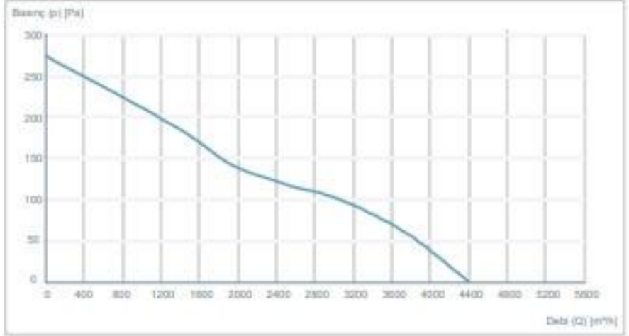
CTAXI 450-5-25
