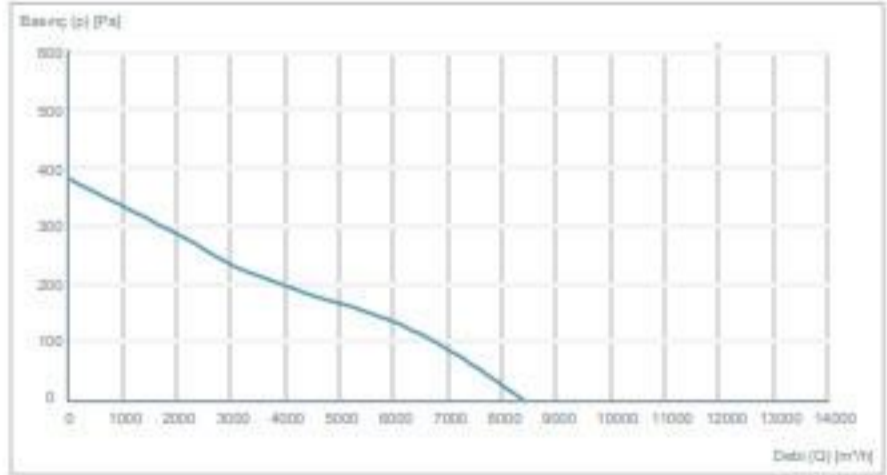
CTAXI 560-5-25
