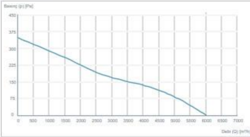
CTAXI 500-5-25
