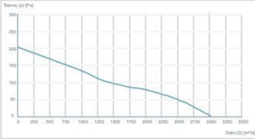
CTAXI 400-5-25
