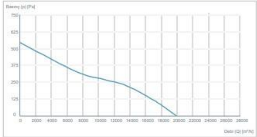
CTAXI 710-5-30
