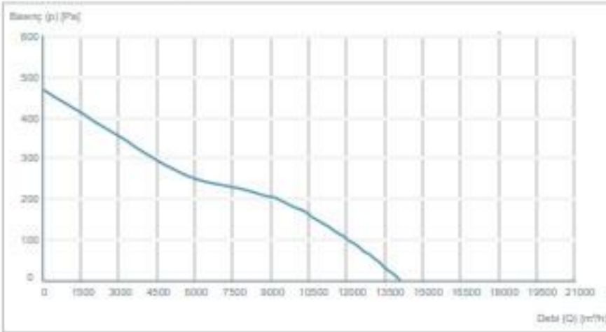
CTAXI 630-5-30
